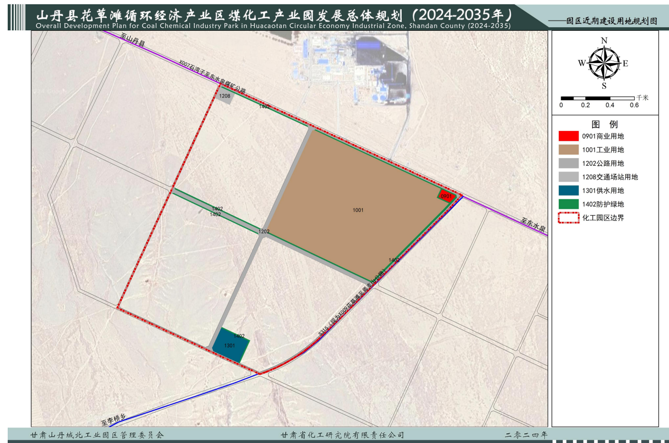
图 5-2 花草滩循环经济产业区煤化工产业园近期建设用地规划图
