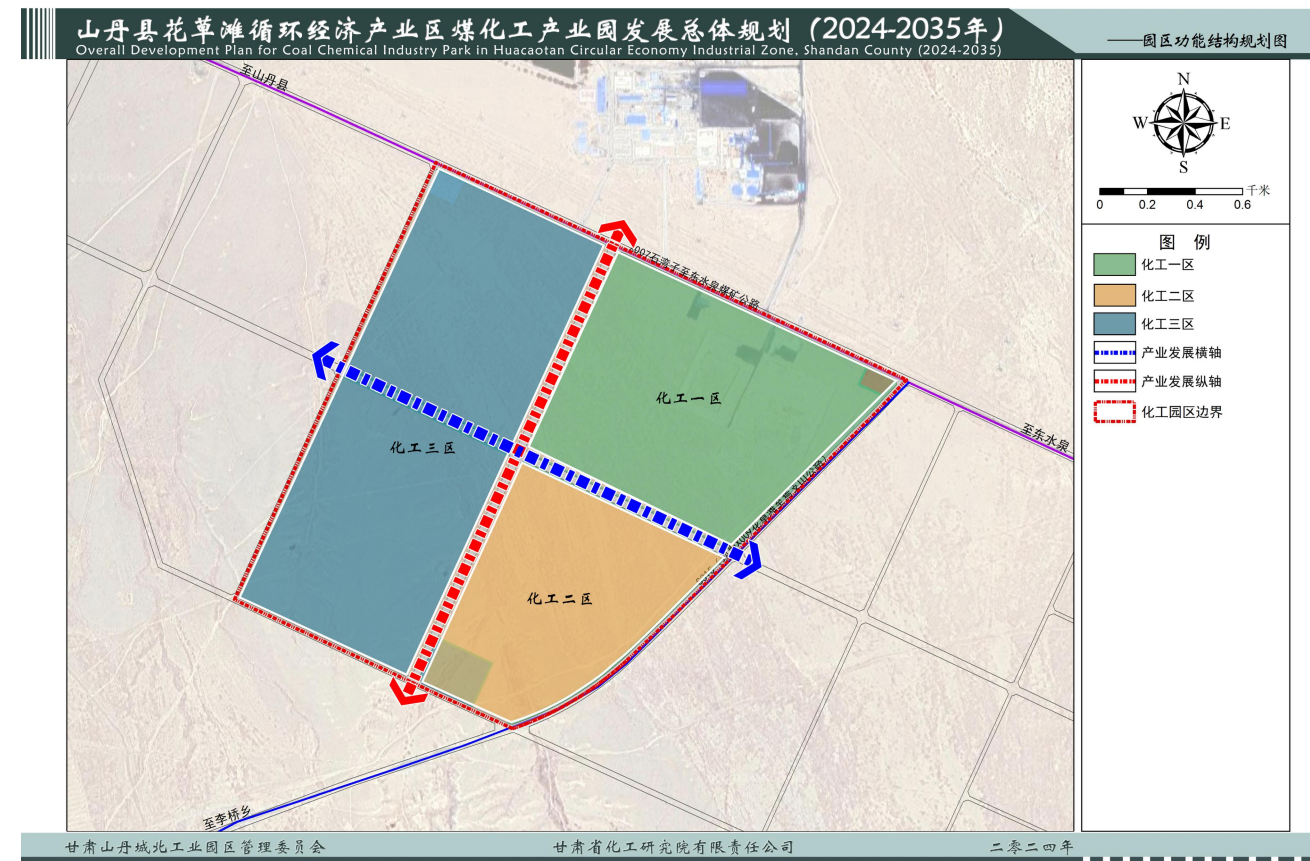
图 5-1 花草滩循环经济产业区煤化工产业园产业功能分区规划图
