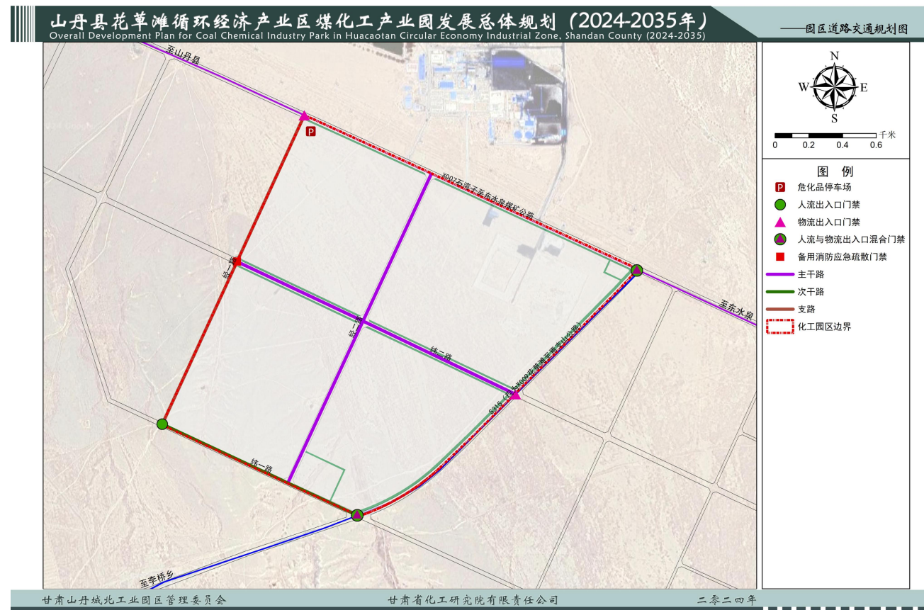
图 6-1 花草滩循环经济产业区煤化工产业园道路交通规划图
