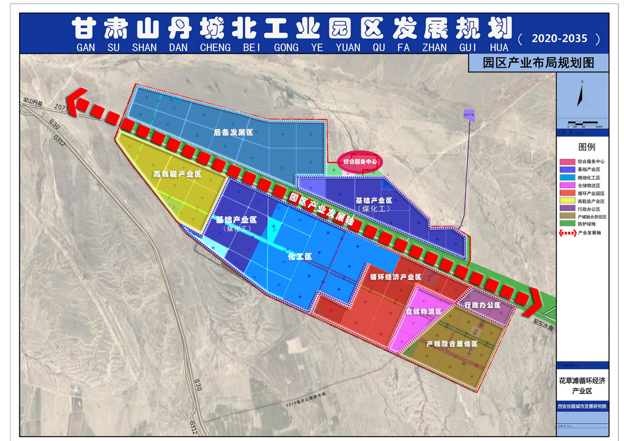
图 1-1 《甘肃山丹城北工业园区发展规划（2020—2035）》花草滩循环经济产业区产业布局规划图
