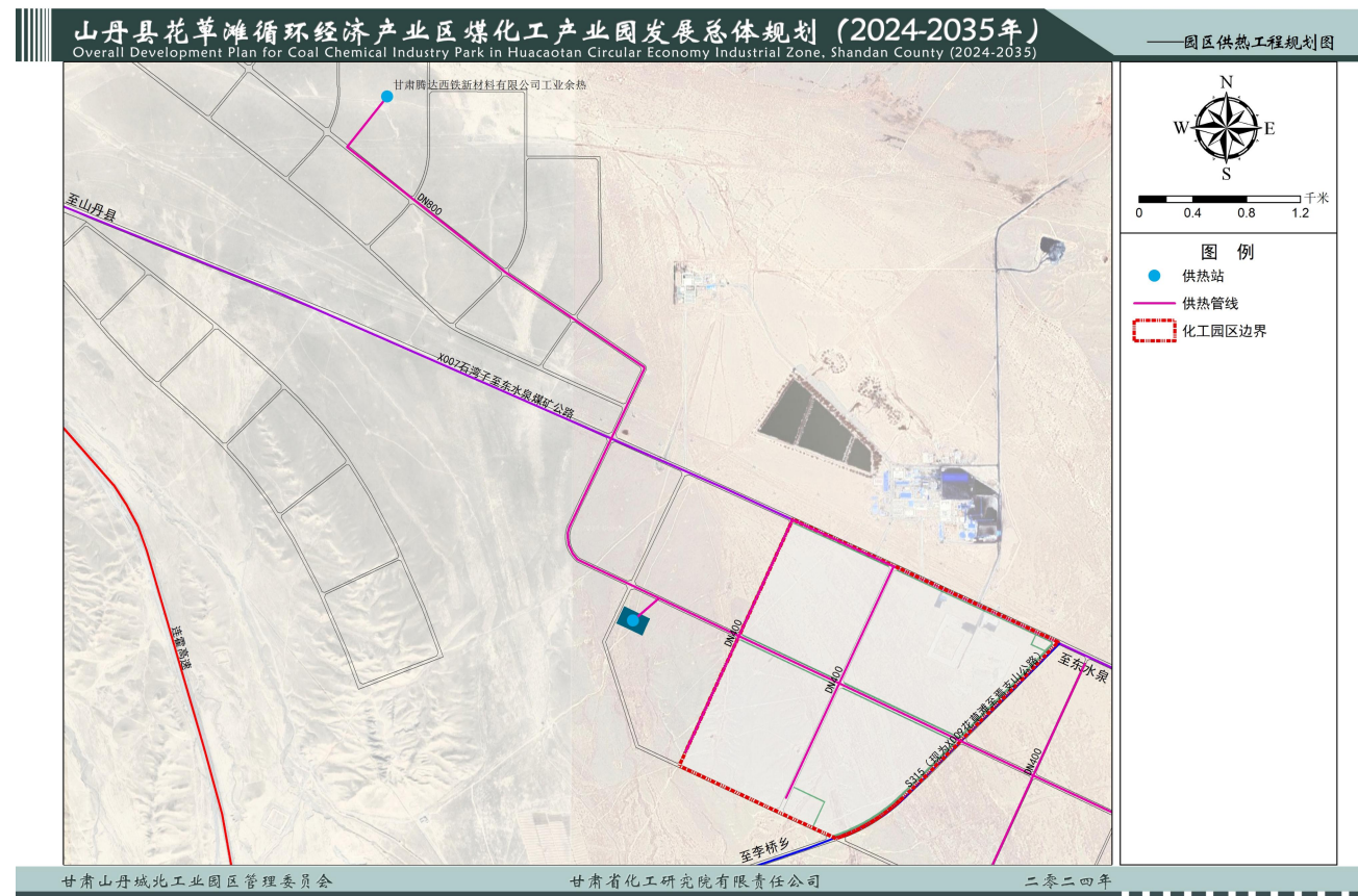
图 9-7 花草滩循环经济产业区煤化工产业园供热及蒸汽工程规划图
