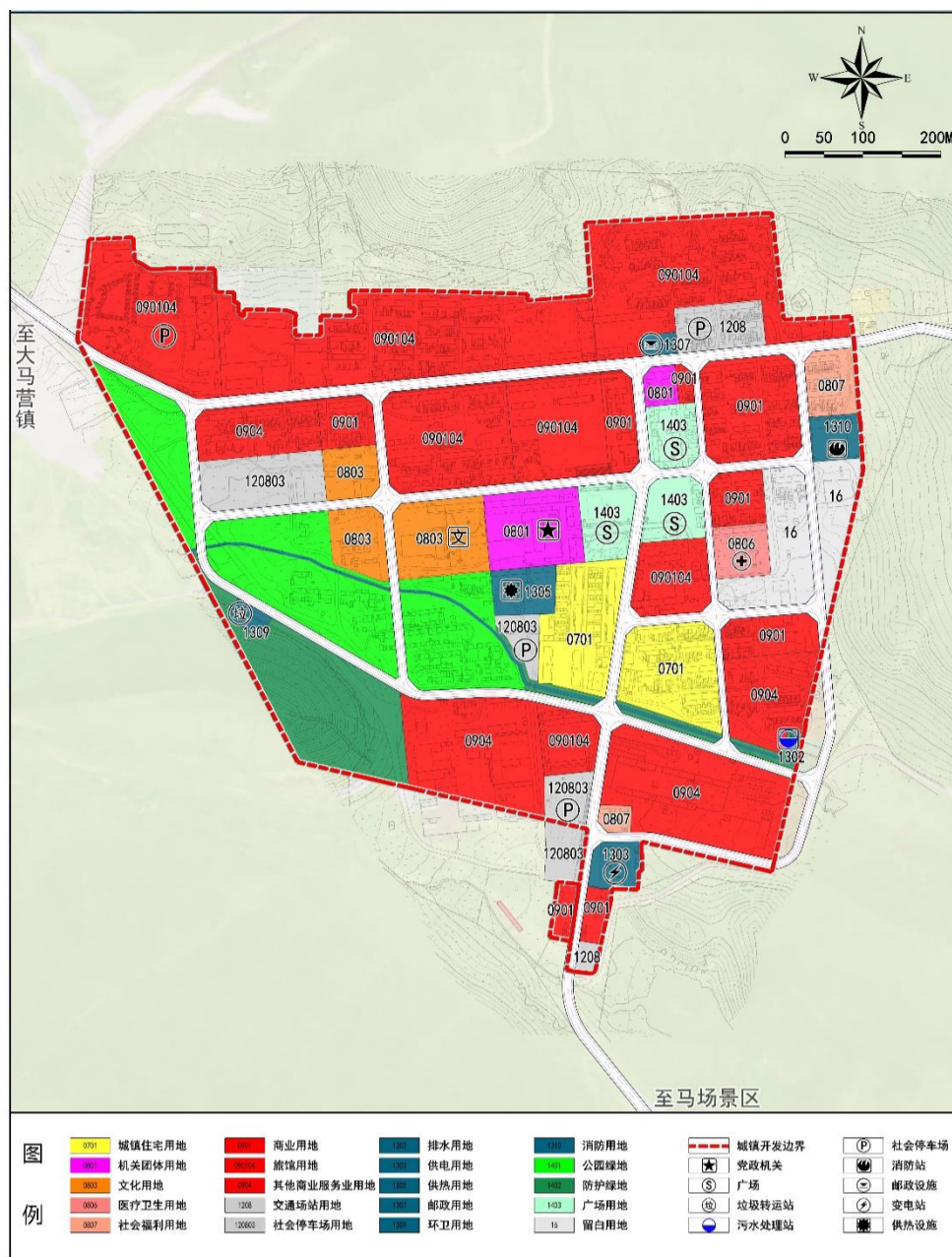
一场国土空间用地规划图
